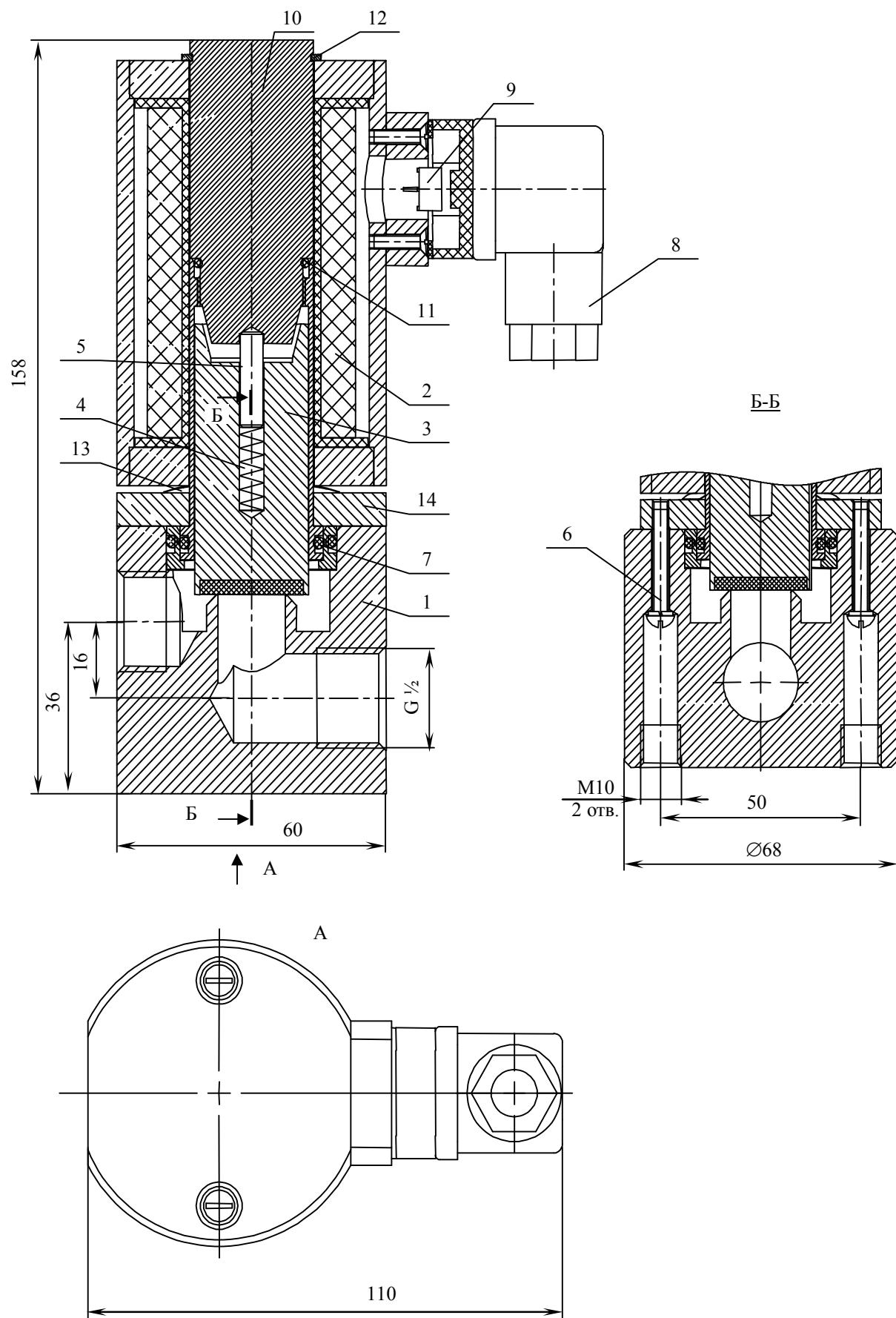
Рис. 1. Устройство клапана ЭМКГ8-15-1-XXX-а304Е.
